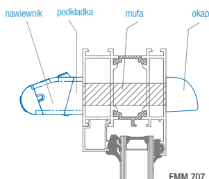
okno aluminiowe – nawiewnik EMM z okapem standardowym i mufą montażową MTM
