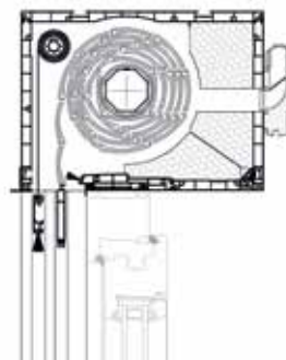
montaż nawiewnika EAH w kasce rolety nadstawnej OpoTerm
